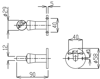
ブラケット詳細
