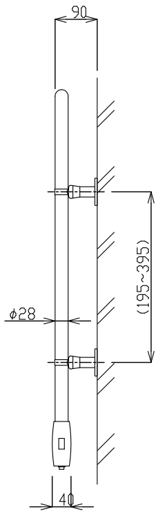
側面(共通)
