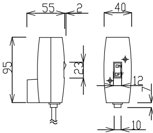
スイッチボックス詳細
